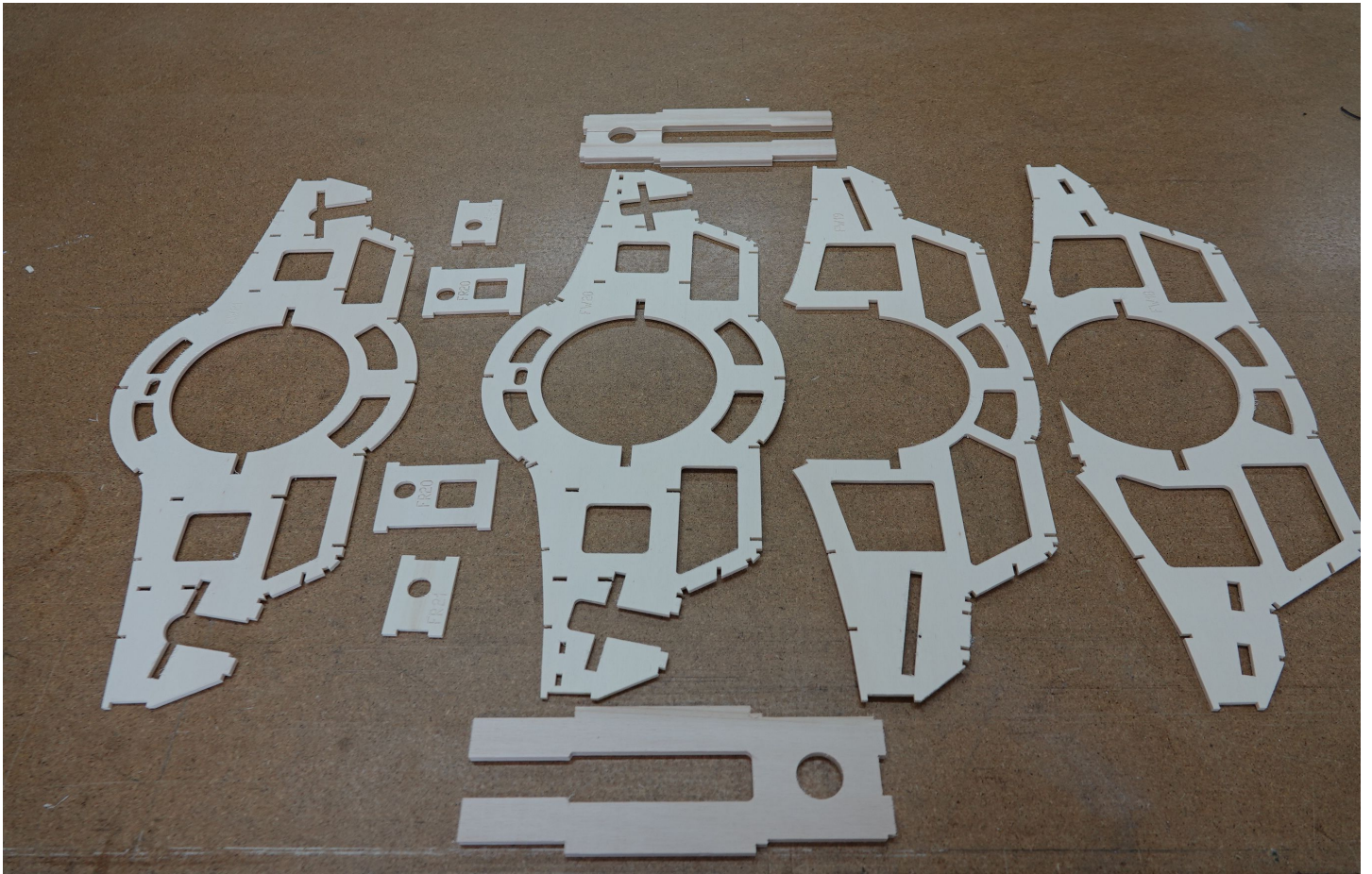
FW18, FW19 Teil nicht nach Plan, FW20, FW21, FR20, FR21, M4
