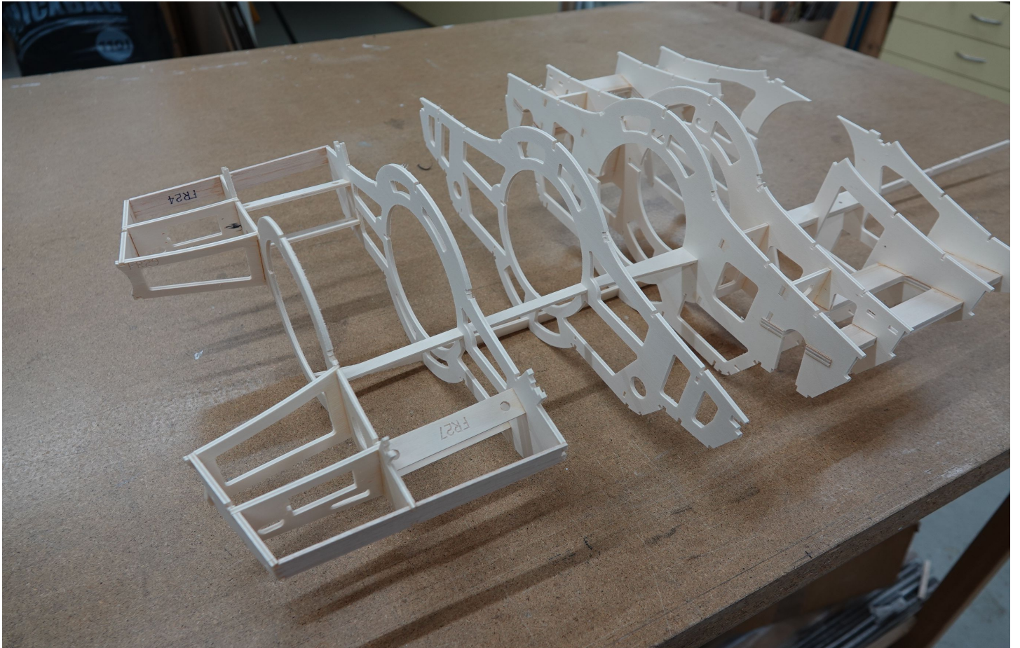
F35A Rumpf hinten
