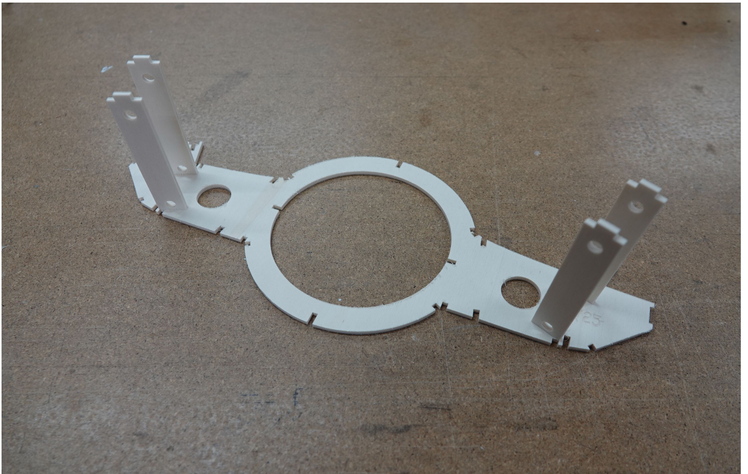
FW25, FR27 und FR28 sind Identisch auf richtige Position der Löcher achten
